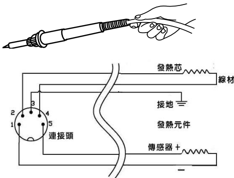
引线示意图
